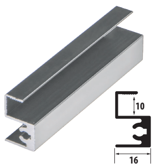
Профиль горизонтальный верхний
