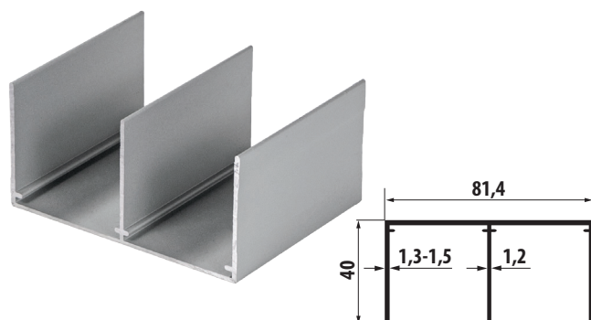
Направляющая верхняя STANDART
