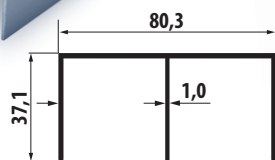
Направляющая верхняя двухполосная ECO
