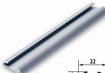
Направляющая для распашной двери
